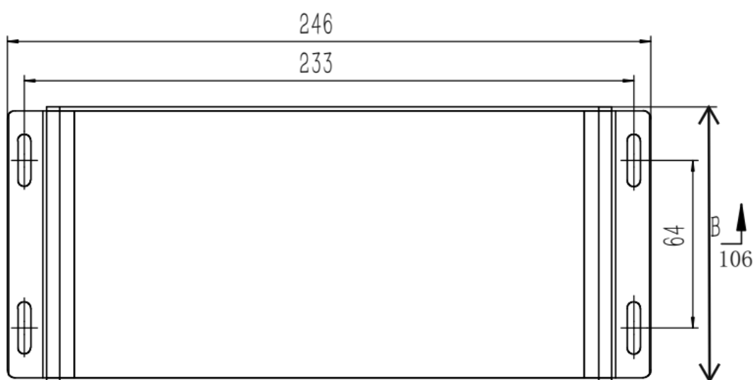
图 2-2 产品尺寸
